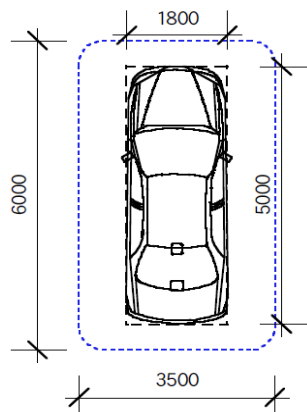
車両寸法例
